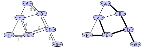
(a) Construcción paso a paso del árbol de recubrimiento (E es el nodo central)
