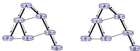
(a) Difusión iniciada en A
